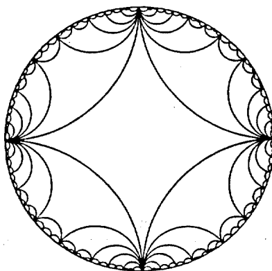
(d) [4, \infty]
