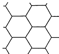
(c) [6, 3]
